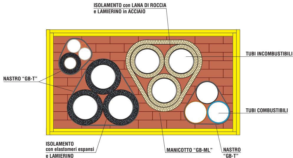
ATTRAVERSAMENTO MULTIPLO VALIDO ANCHE IN PRESENZA DI TUBI INCOMBUSTIBILI COIBENTATI E NON (vedi pag 164)
