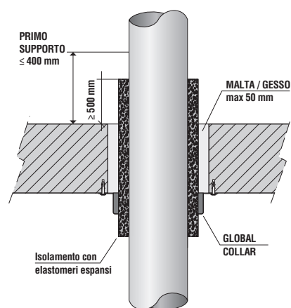
TUBO CON ISOLAMENTO con elastomeri espansi
