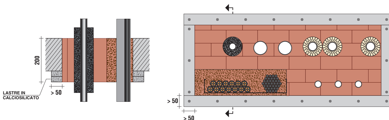
SEZ. SOLAIO CON SPESSORE COMPRESO TRA 150 E 200 mm con GLOBAL BLOCK lato 200 mm in altezza e schiuma GLOBAL FOAM Comice con doppia lastra in calciosilicato di larghezza 50 mm
