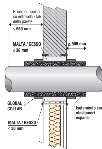
TUBO CON ISOLAMENTO con elastomeri espansi
