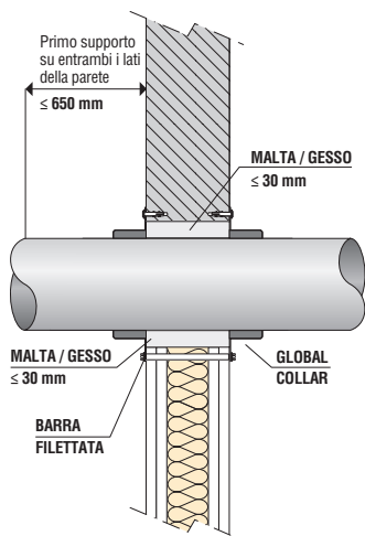
TUBO SENZA ISOLAMENTO
