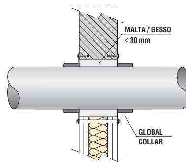
TUBO CON ISOLAMENTO con elastomeri espansi
