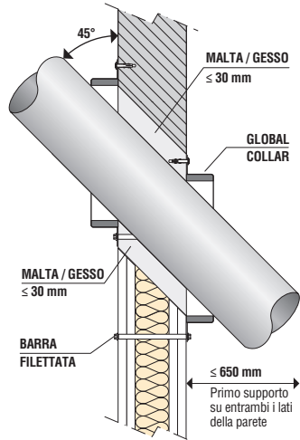
TUBO SENZA ISOLAMENTO inclinazione massima 45°
